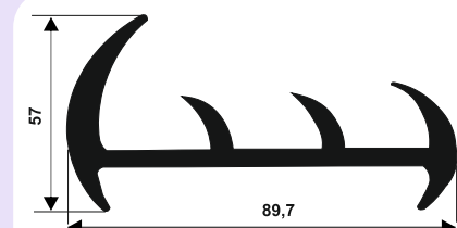
087 KAUÇUK CONTA
