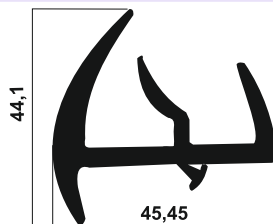
088 KAUÇUK CONTA
