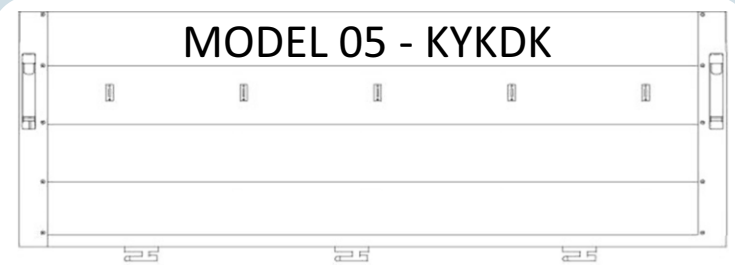
KANCALI YAN KAPAK DİK KİLİT B=80 CM
