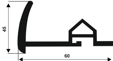
083 KAUÇUK CONTA
