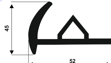
086 KAUÇUK CONTA
