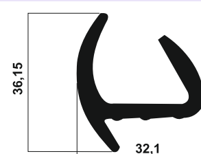
090 KAUÇUK CONTA
