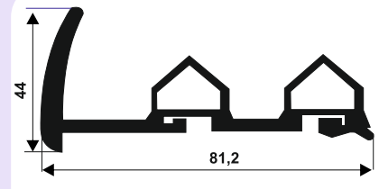
084 KAUÇUK CONTA
