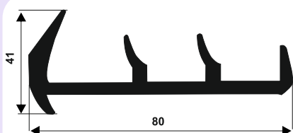
085 KAUÇUK CONTA
