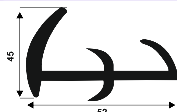
089 KAUÇUK CONTA
